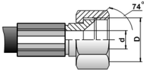
DKI-(Г) фитинг с накидной гайкой
