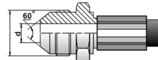
JIS-(Ш) ниппель с наружной резьбой
